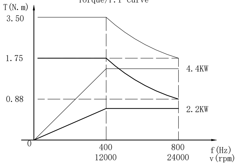
扭矩/功率曲线
