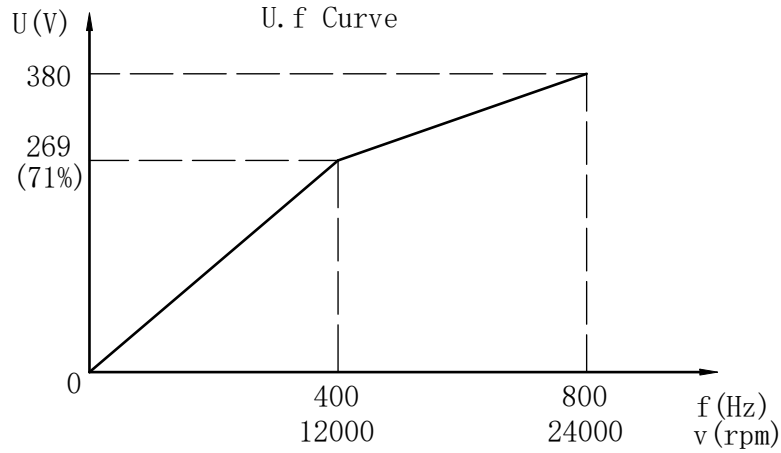
频压曲线
